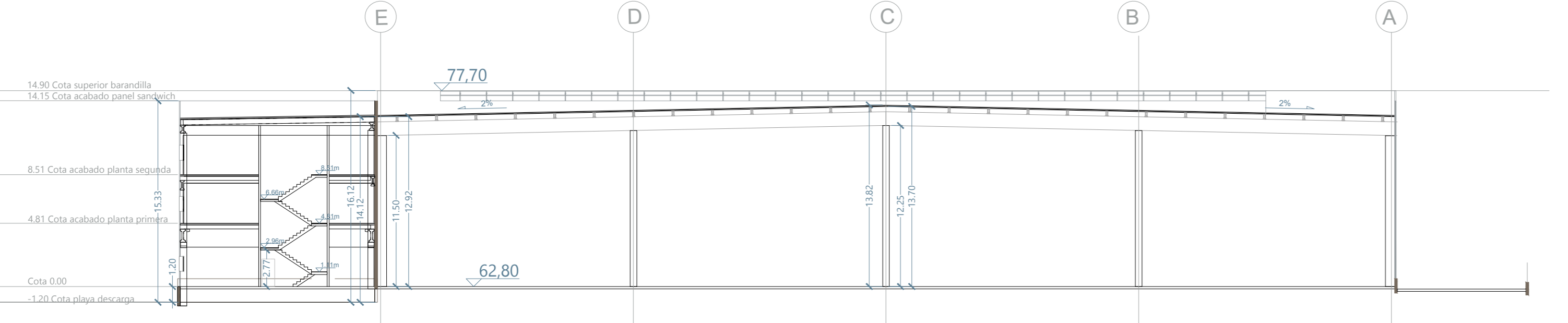
SECCIÓN TRANSVERSAL C-C' Escala 1:300
