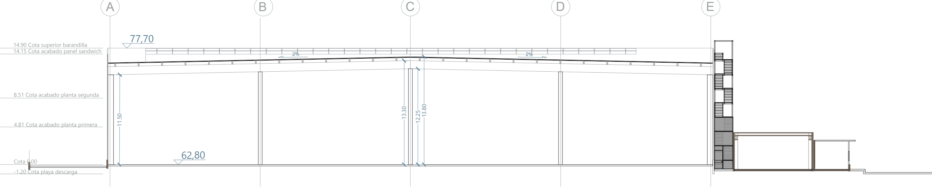
SECCIÓN TRANSVERSAL B-B' Escala 1:300
